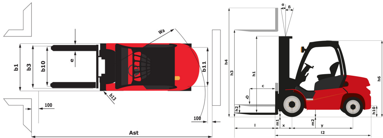
MI 18 G ST5 - Schémas d'encombrement
