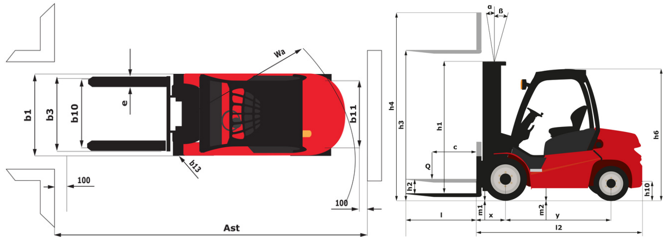
MI 25 D ST5 - Schémas d'encombrement
