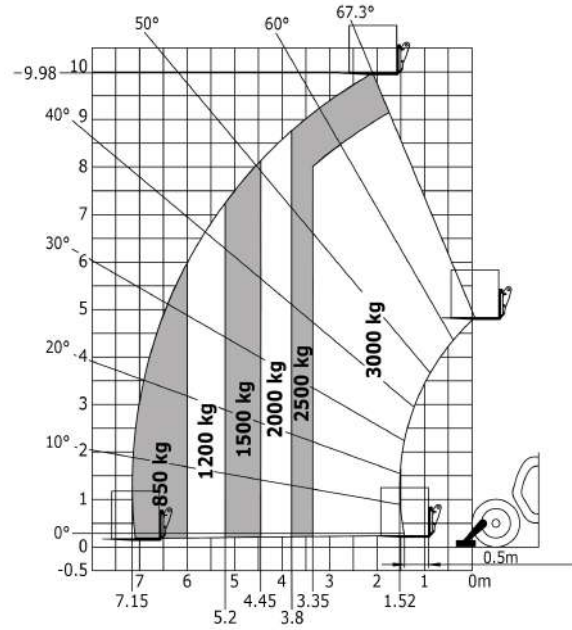
Rotation sur stabilisateurs déployés avec fourches
